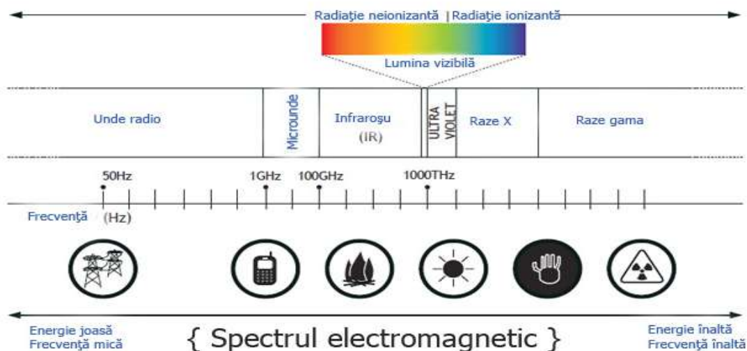
Figura nr. 64 Spectrul electromagnetic
