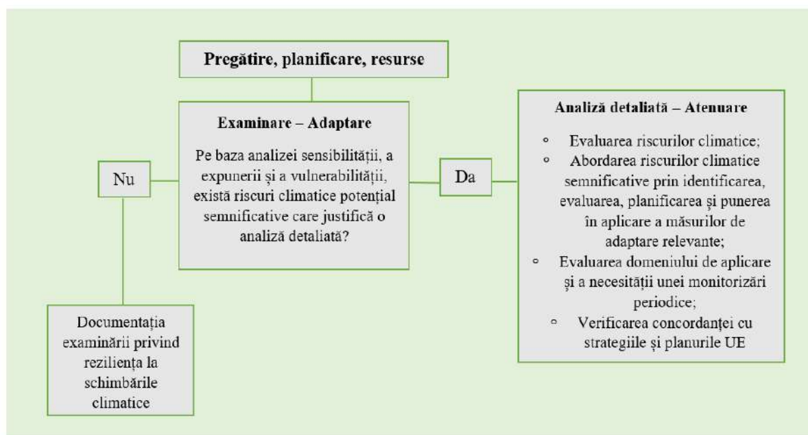
Figura nr. 65 Prezentare generală a procesului de adaptare la schimbările climatice pentru imunizarea la schimbările climatice
