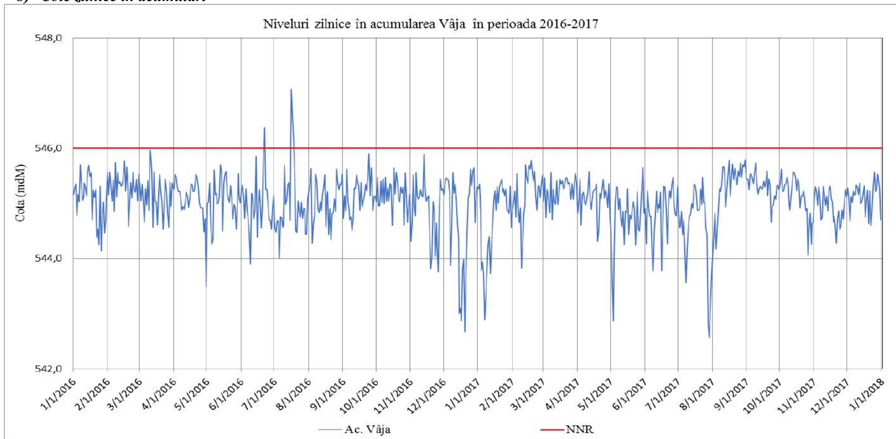
Figura nr. 7 Exemplu de niveluri zilnice în acumularea Vâja în perioada 2016-2017
